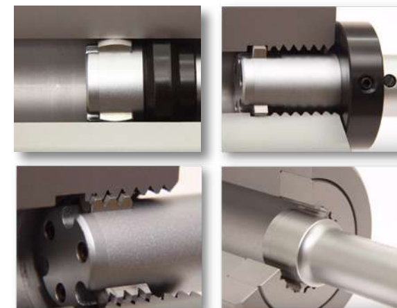
Głowice specjalne do rowków, gwintów, wielowypustów itp. dostępne na zapytanie
