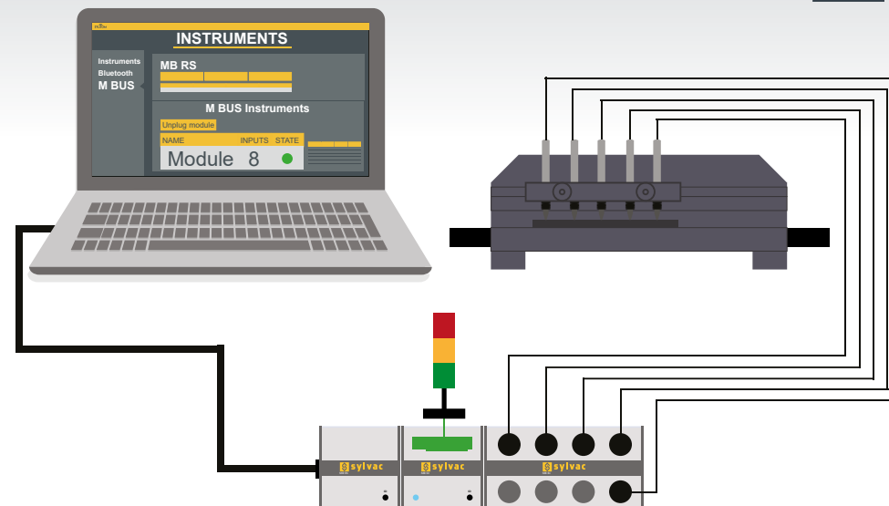
Moduł główny M-Bus RS umożliwiający połączenie różnych modułów do PC
